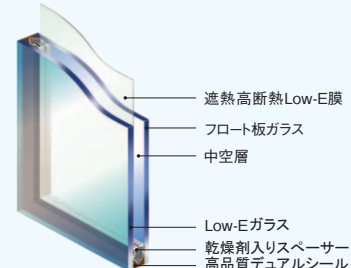
遮熱低放射複層ガラス ペアマルチEAグリーン
