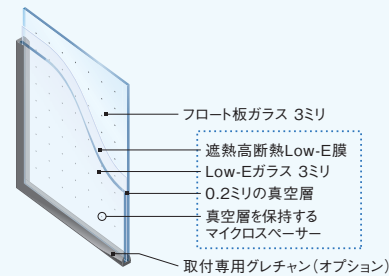
真空ガラス スペースシアクール
