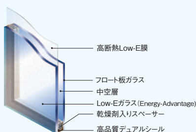
低放射複層ガラス ペアマルチEA
